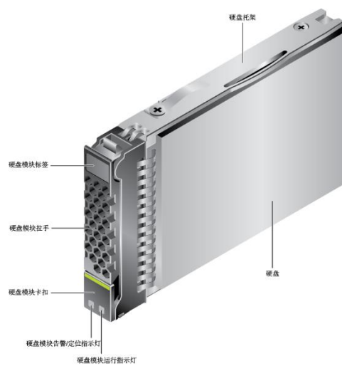
图1-39 硬盘模块
