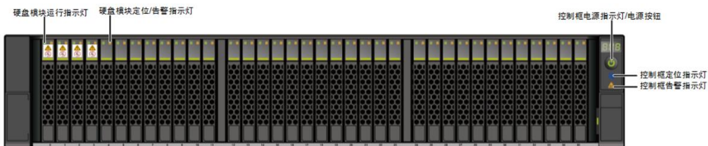
图1-41 2U 36 盘位控制框前面板指示灯
