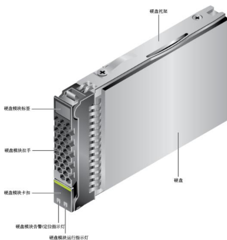
图1-24 硬盘模块
