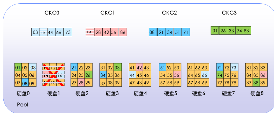
图1-73 RAID2.0+快速重构示意图（一）
