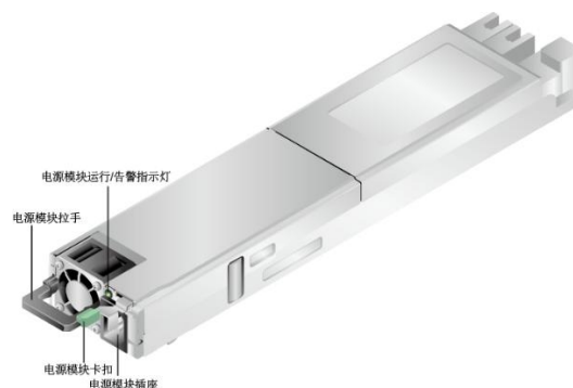
图1-68 交流电源模块
