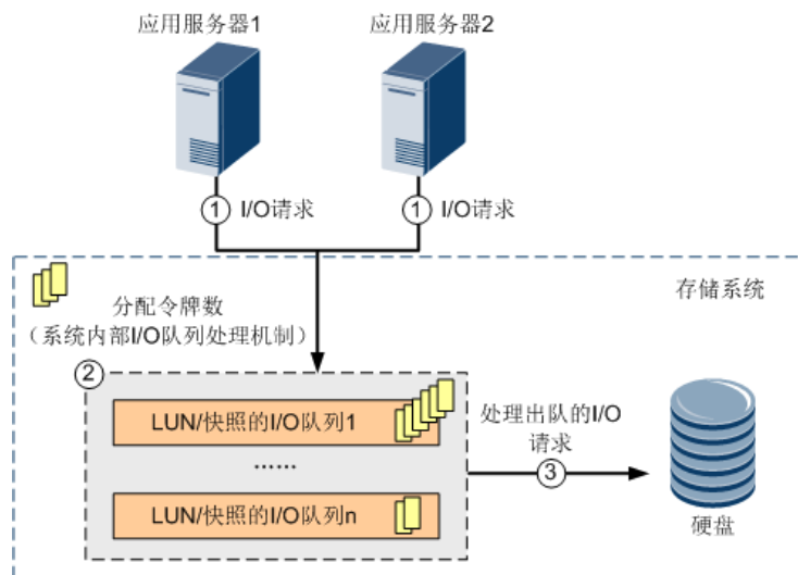
图1-82 基于 LUN 或快照的 I/O 流量控制队列管理
