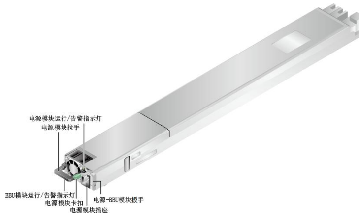
图1-38 电源-BBU 模块后视图
