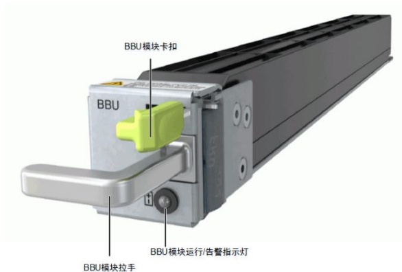
图1-21 BBU 模块前视图
