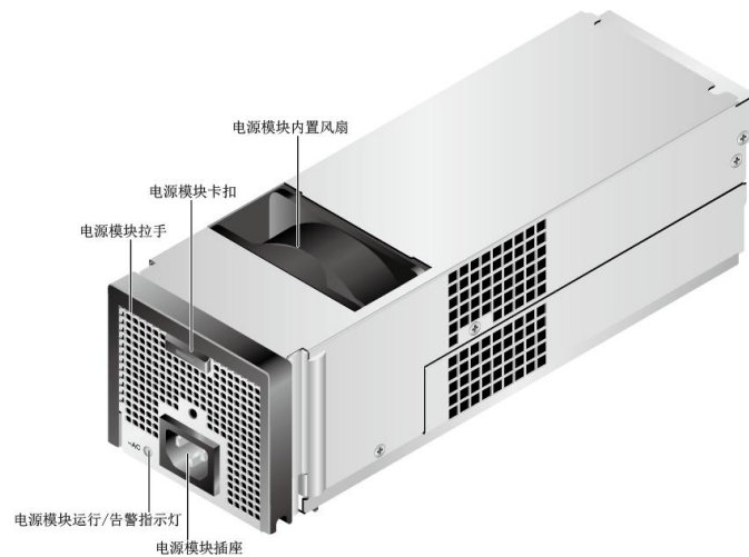
图1-64 交流电源模块
